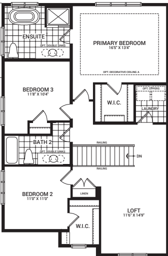
OPTIONAL LOFT IN LIEU OF BEDROOM 4
