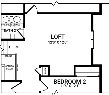
OPTIONAL LOFT IN LIEU OF BEDROOM 4
