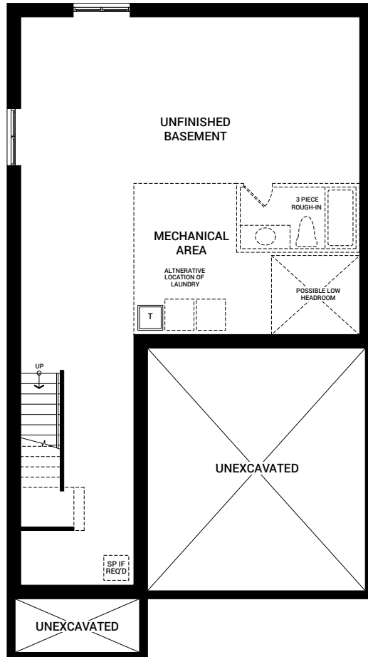
BASEMENT PLAN A, B, C & D
