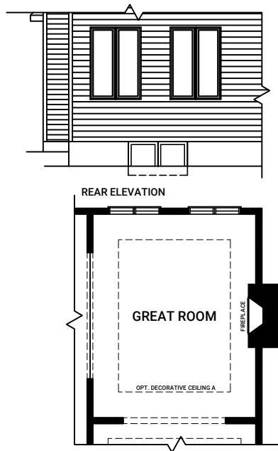
OPTIONAL IN-OUT FIREPLACE
