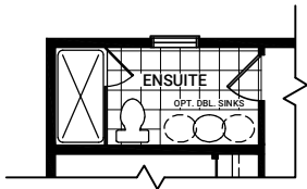
ENSUITE OPTIONAL 1 WALL SEAMLESS SHOWER
