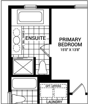
OPTIONAL ENSUITE LAYOUT A
