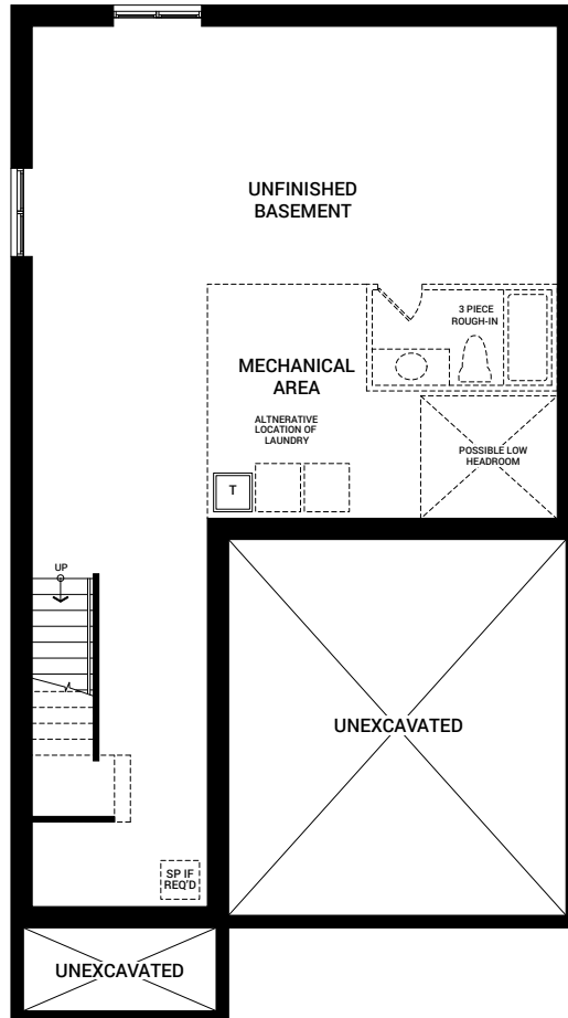
BASEMENT PLAN A, B, C & D
