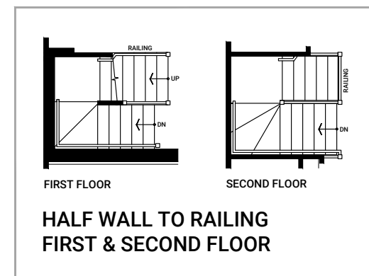
STAIR OPTIONS
