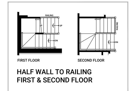
STAIR OPTIONS
