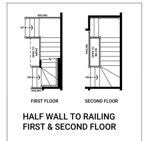
STAIR OPTIONS
