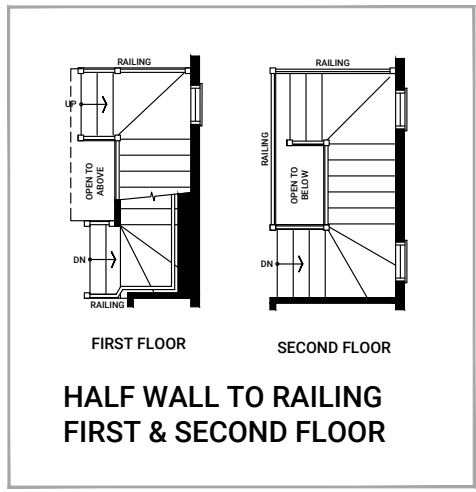
STAIR OPTIONS
